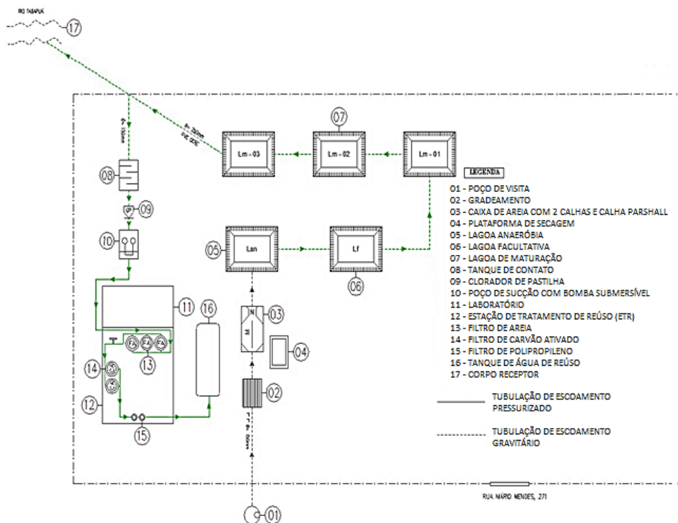
Figura 1 – Descrição do Sistema de Tratamento de Esgoto da Estação Guadalajara
