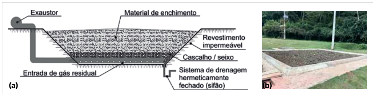
Figura 6 – Biofiltro não estruturado com enchimento de fundo: a) desenho esquemático; b) foto em uma ETE.
