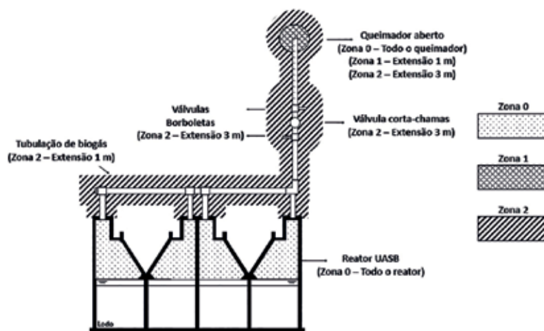
Figura 5 – Mapa esquemático das zonas de riscos de explosão em uma ETE com reator anaeróbio.
