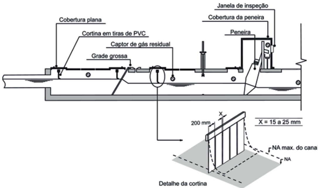
Figura 3 – Esquema da contenção de odores e gases corrosivos no tratamento preliminar.
