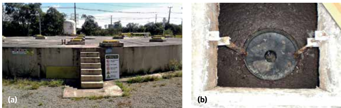
Figura 3 – Sistema inexistente e/ou ineficiente de remoção de espuma: a) reator anaeróbio sem dispositivo de remoção de espuma; b) abertura da tampa de inspeção para remoção de espuma.
