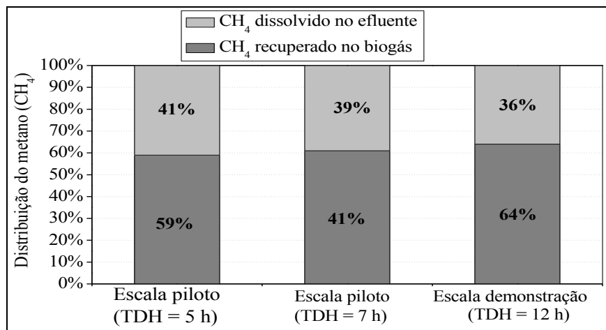
Figura 4 – Perdas de CH 4 dissolvido em efluente de reatores UASB e recuperado no biogás.
