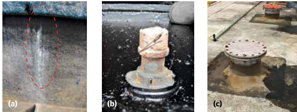
Figura 1 - Ilustração de pontos de ocorrência de vazamentos de biogás: a) Fissura presente no STF de reator UASB; b) Conexão da tubulação de biogás danificada; c) Vazamento de gás em inserts no concreto.
